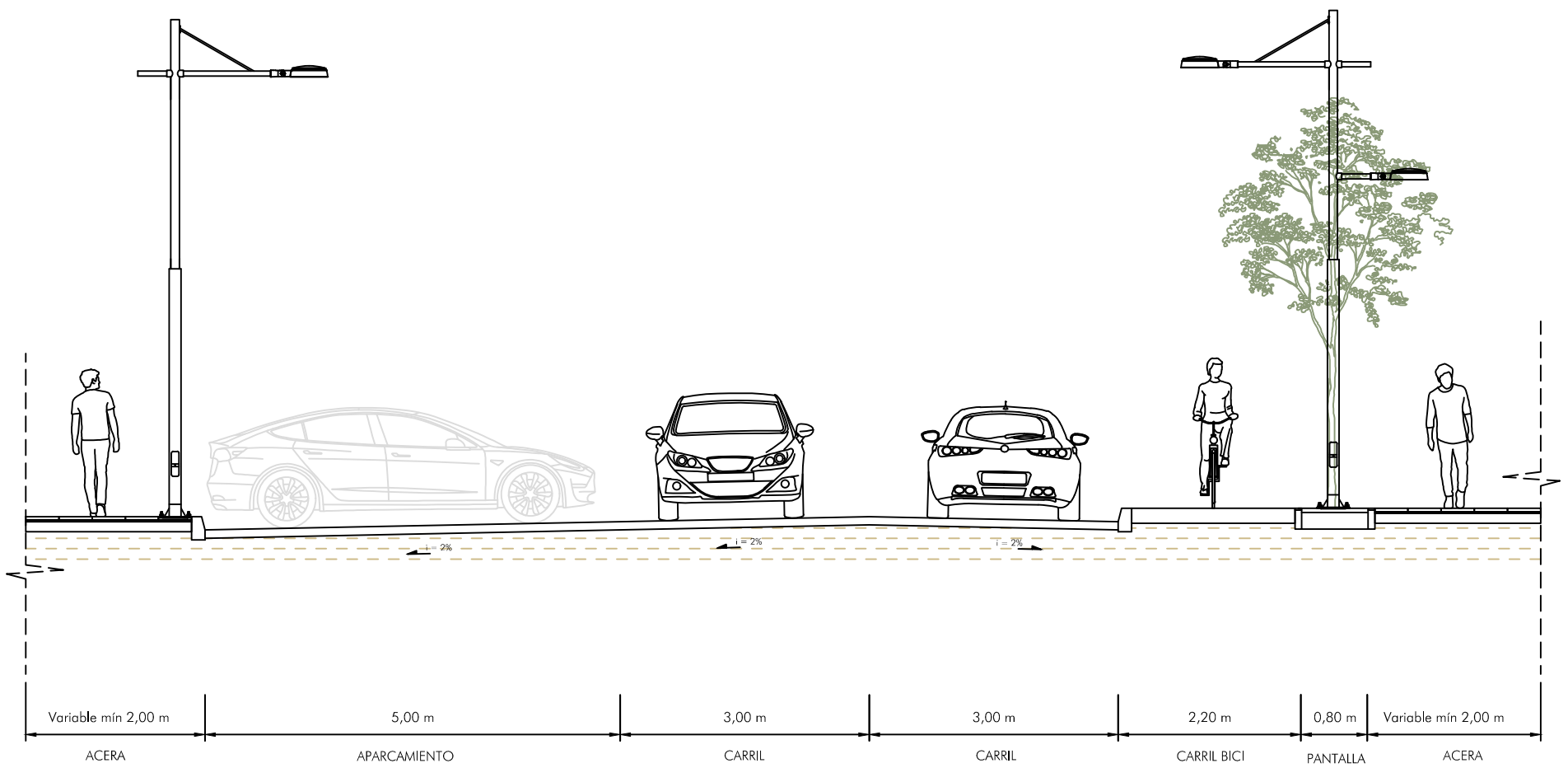
SECCIÓN TIPO RESIDENCIAL (II)
